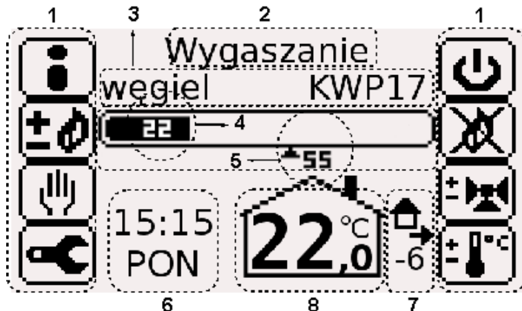
Rys.1. Widok panelu sterowania i ekranu głównego wyświetlacza.
